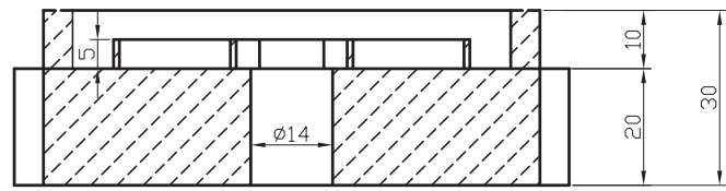
VIEW A-A
